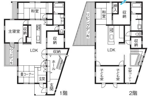
間取り図
